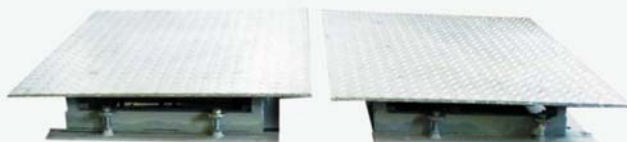
Испытательные площадки перемещаются гидроприводом
